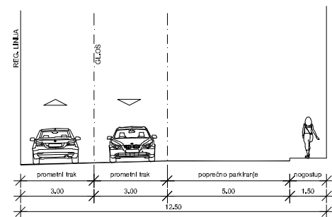
POPREČNI PRESJEK "A"
