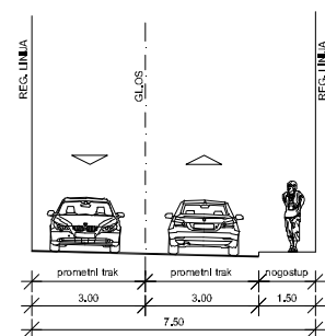
POPREČNI PRESJEK "B"
