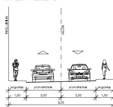
POPREČNI PRESJEK "B"
