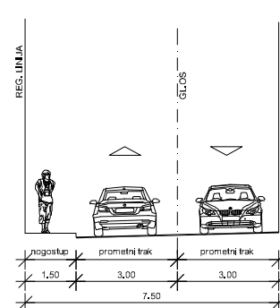
POPREČNI PRESJEK "A"
