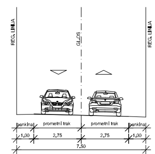
POPREČNI PRESJEK "A"
