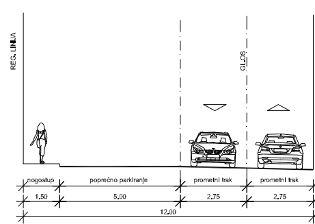
POPREČNI PRESJEK "B"
