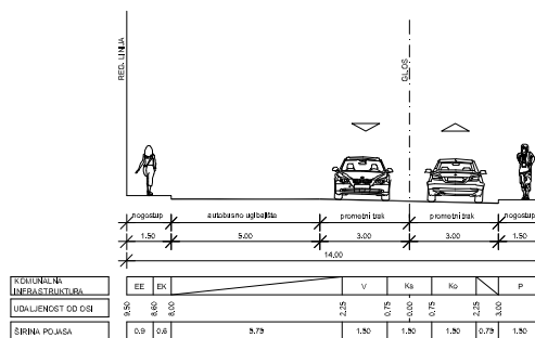
POPREČNI PRESJEK "A"
