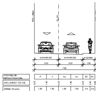
POPREČNI PRESJEK "B"
