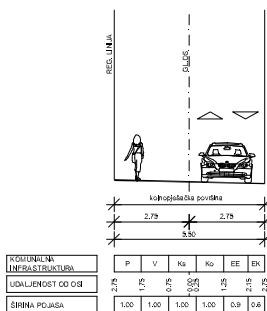
POPREČNI PRESJEK "C"
